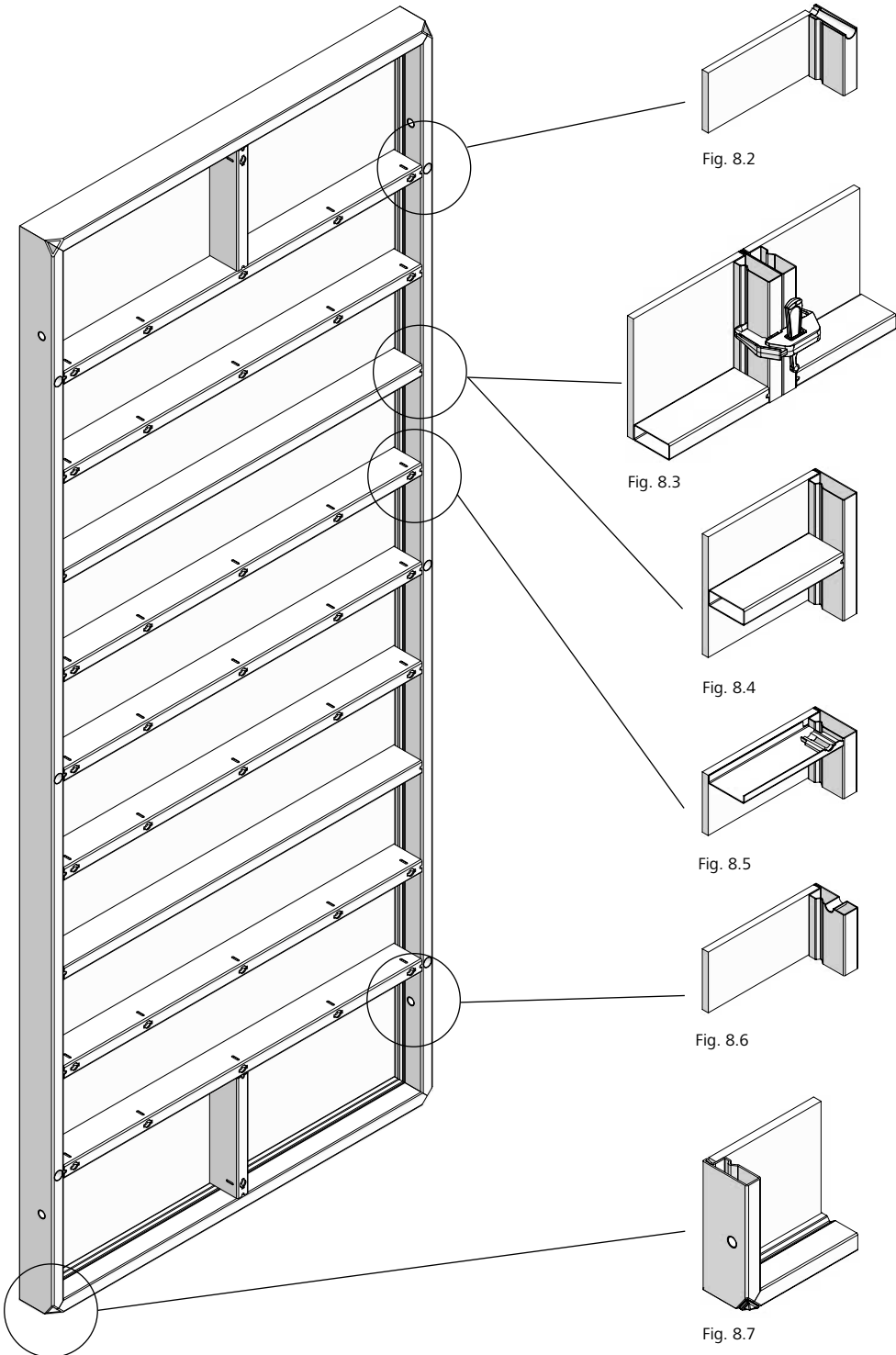
Fig. 8.1 StarTec 330/135
