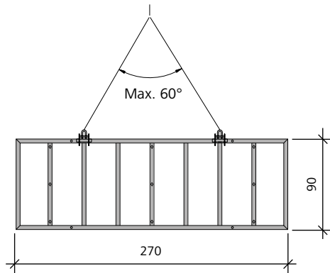
Fig. 60.1 AluStar/StarTec
