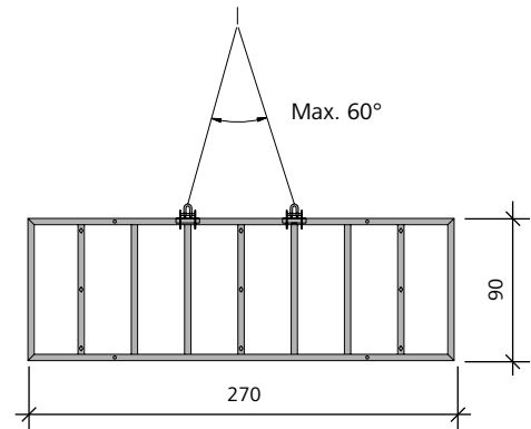
Fig. 60.2 AluStar/StarTec
